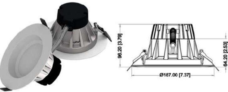
MOD: LLUL-CDL6S-912W-ES-4 6inch 12W 1050lm
